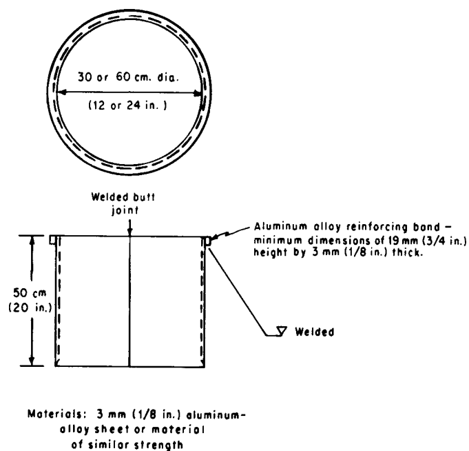
FIG. 1 Infiltrmeter Construction
